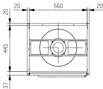
EC Radial Fan
