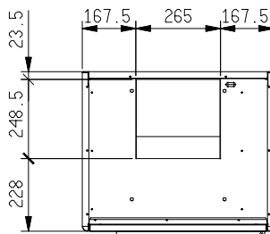
Centrifugal Fan
